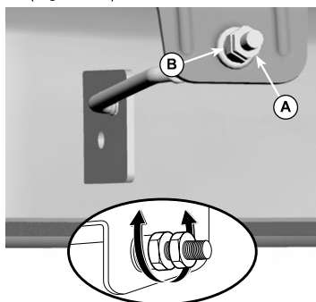
Fig. 26 – Porca de ajuste
