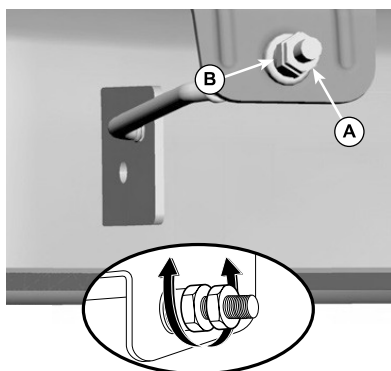
Fig. 26 – Tuerca de ajuste
