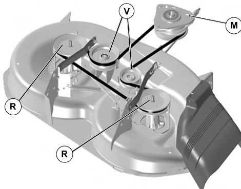
Fig. 27 – Instalación de la correa motora
