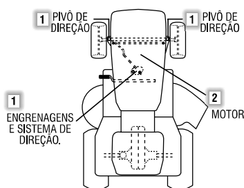
Fig. 14 – Pontos de lubrificação
