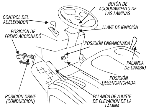
Fig. 11 – Ajuste del freno de estacionamiento
