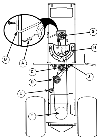
Fig. 28 – Sustituir la correa
