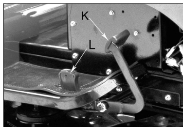
Fig. 5 – Pedales de aceleración
