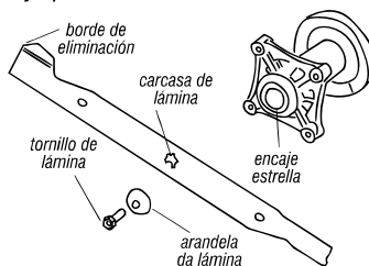
Fig. 15 – Lámina de corte
