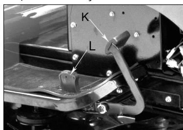
Fig. 5 – Pedais de aceleração
