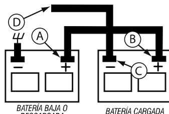
Fig. 30 – Cable de transmisión/puente
