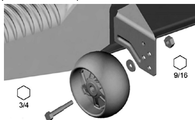
Fig. 6 – Rodas niveladoras
