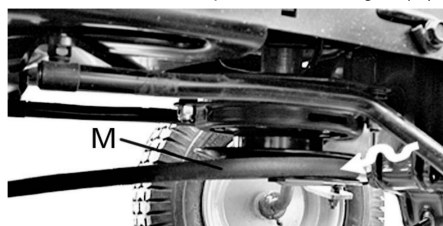
Fig. 22 – Correa e polea da embreagem
