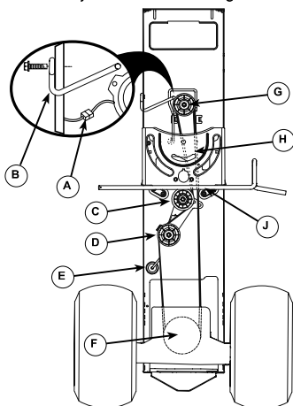
Fig. 28 — Substituir a correia
