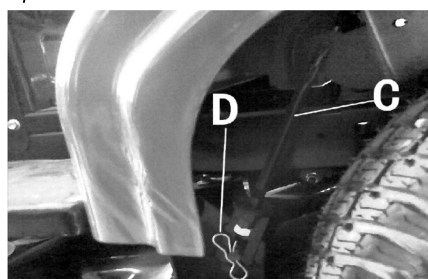
Fig. 20 – Elevador trasero
