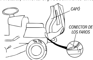
Fig. 31 – Remover capó
