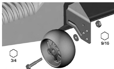
Fig. 6 – Ruedas niveladoras
