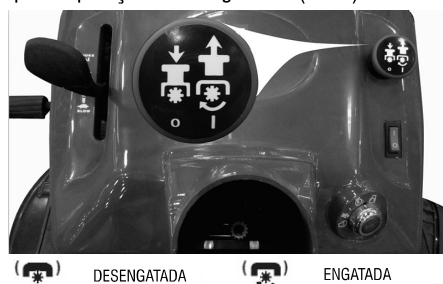
Fig. 3 – Acionamento das lâminas de corte
